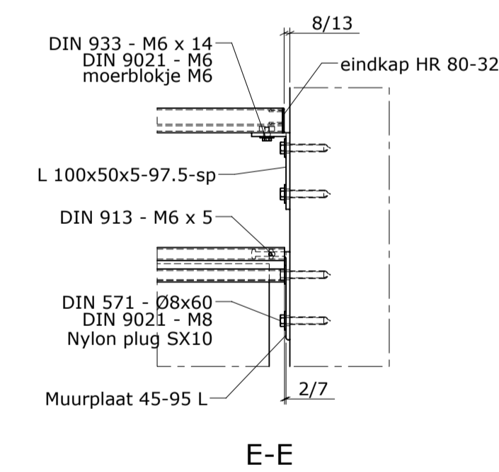
E-E
